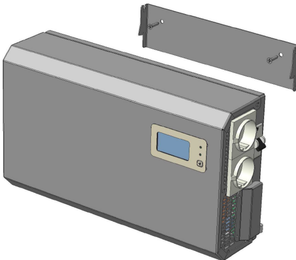
Рисунок 3.1 - Крепление стабилизатора к стене
